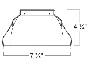
PRLK-600 (6")
